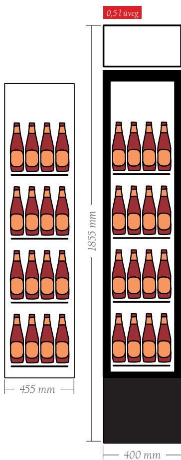
Felépítmény méretek
