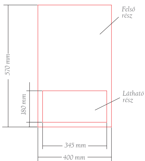
Felépítmény méretek
