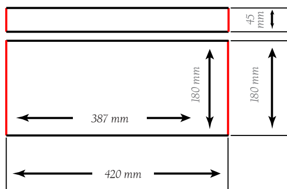
Felépítmény méret
